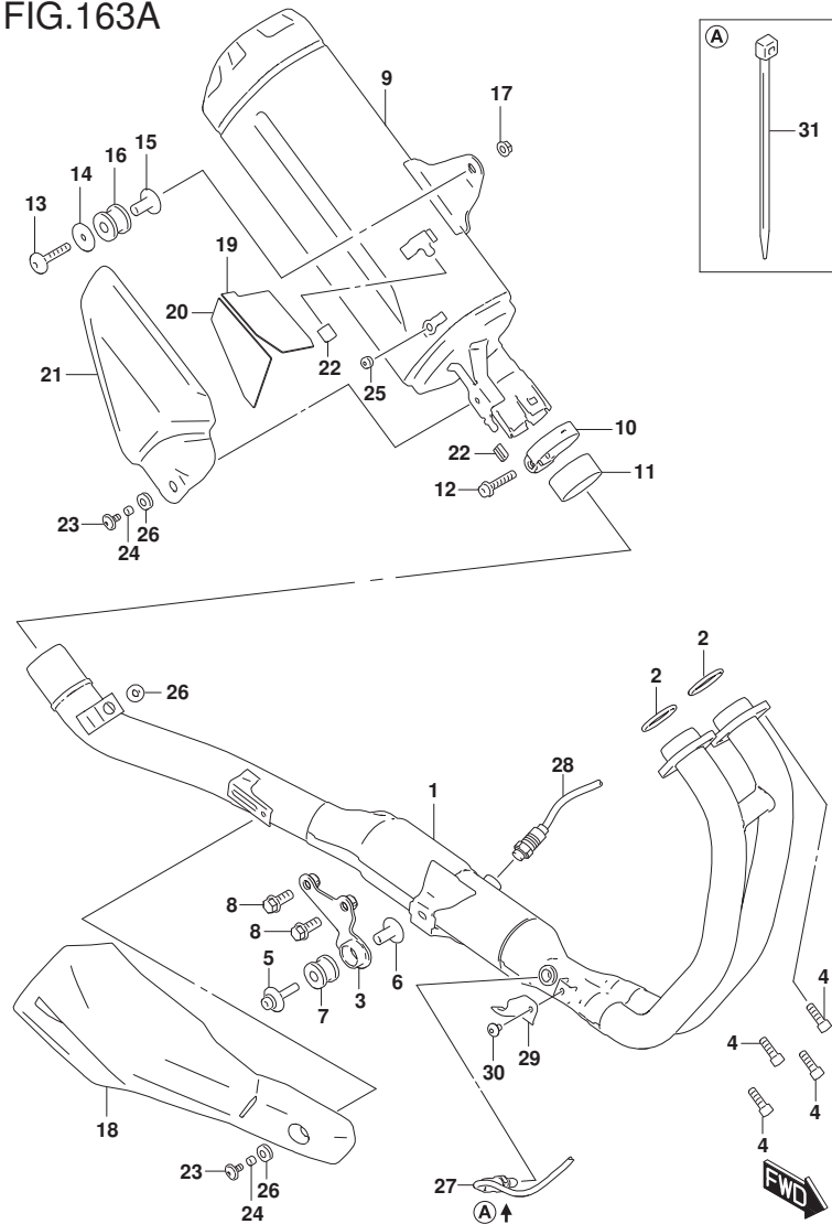
FIG.163A (1-C-5) MUFFLER
