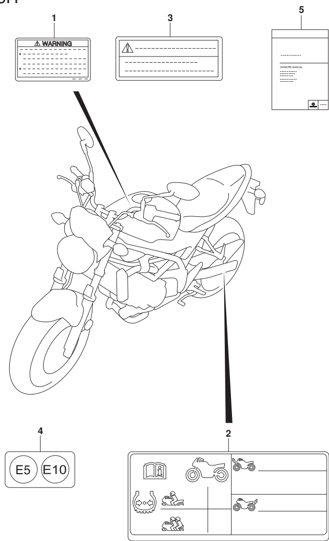
FIG.496H (2-C-13) LABEL (SV650XAU9 E19)
